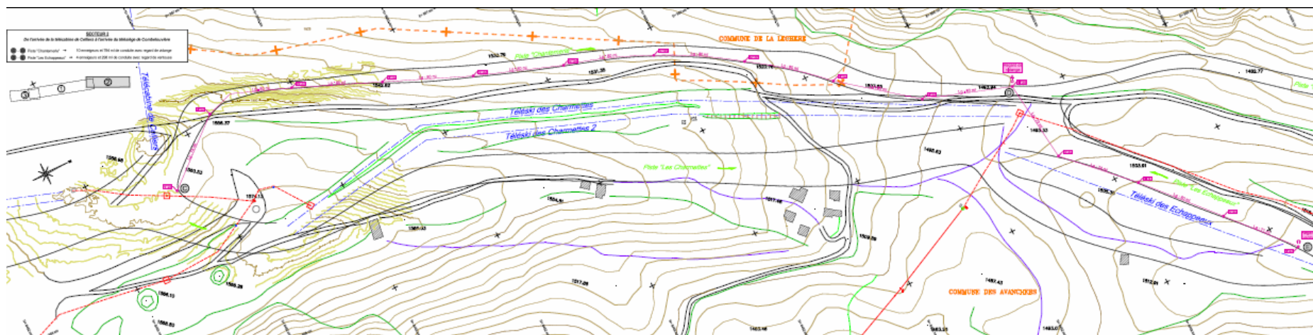
Plan initial du réseau neige de la section 1
