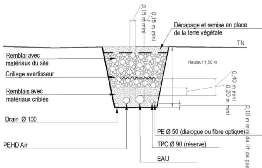
Coupe type réseau neige
